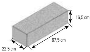
Typ 1: Grundelement groß Sichtflächen feingestrahlt, Köpfe unbeebeitet, Oberseite feingestrahlt
