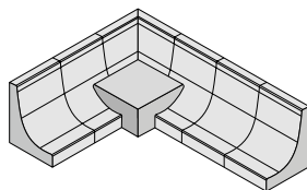
Aufbeton aus Magerbeton C12/15 bei zweiteiligen Winkelecke-Steinen
