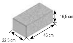
Typ 2: Grundelement klein Sichtflächen feingestrahlt, Köpfe unbeebeitet, Oberseite feingestrahlt
