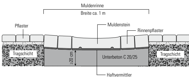
Einbaubeispiel Muldenrinnen
