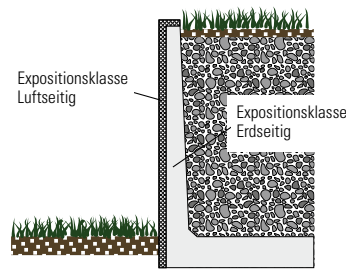
Lage der Expositionsklassen bei KANN Mauerwerk
