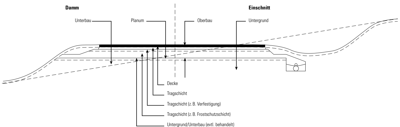
Abb. 3: Beispielhafter Aufbau einer Befestigung außerhalb geschlossener Ortslage sowie in geschlossener Ortslage mit wasser-durchlässigen Randbereichen – Damm/Einschnitt (Aus: Richtlinien für die Standardisierung des Oberbaues von Verkehrsflächen RStO)
